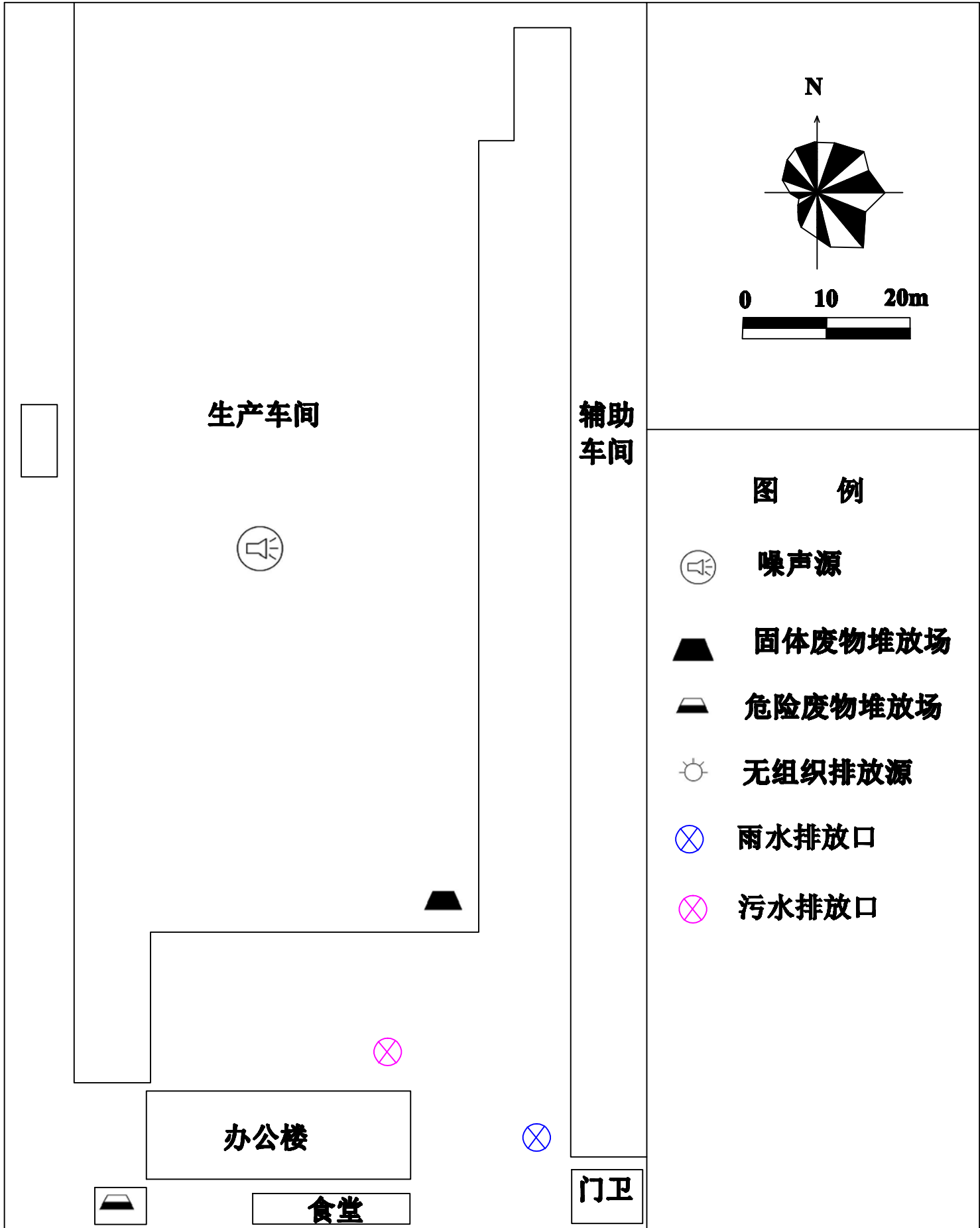
附图3 项目厂区平面布置图
